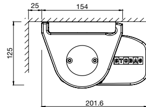
Montage sous dalle
